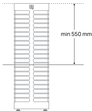
Рисунок 2. Установка каменки HUUM STEEL, частично погруженной в пол.
